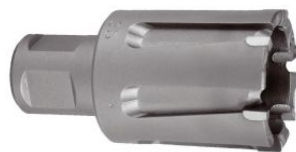
Broca hueca con dientes de Metal Duro y vástago Weldon para vías de tren at.com.es/p/1017934
