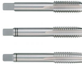
Juego de machos para roscar a mano M DIN 352 HSS rectificados con rosca izquierda
