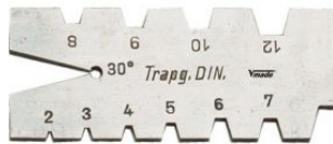
Patrón roscas trapezoidal at.com.es/p/1018270
