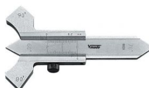
Calibre de precisión para soldaduras
