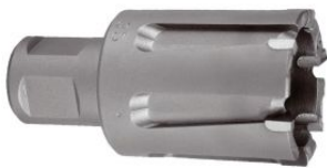
Broca hueca con dientes de Metal Duro y vástago Weldon para vías de tren
